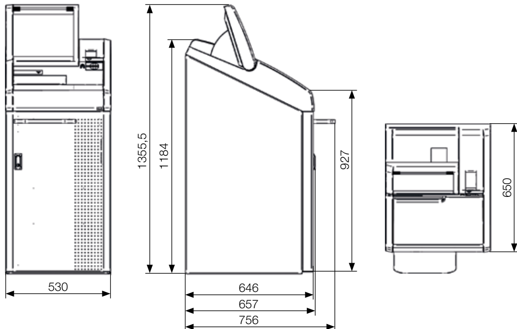
KePlus P6 Kontoauszugsdrucker
